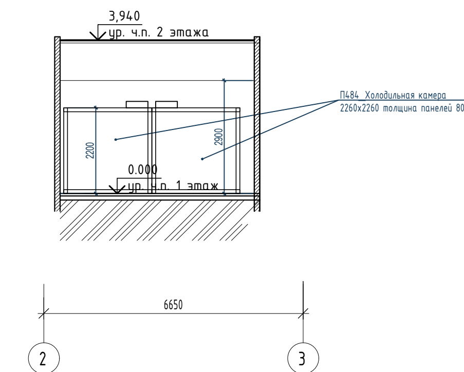
Фрагмент Коридор с местом установки холодильного оборудования пом.14.7.1 разрез 1-1
